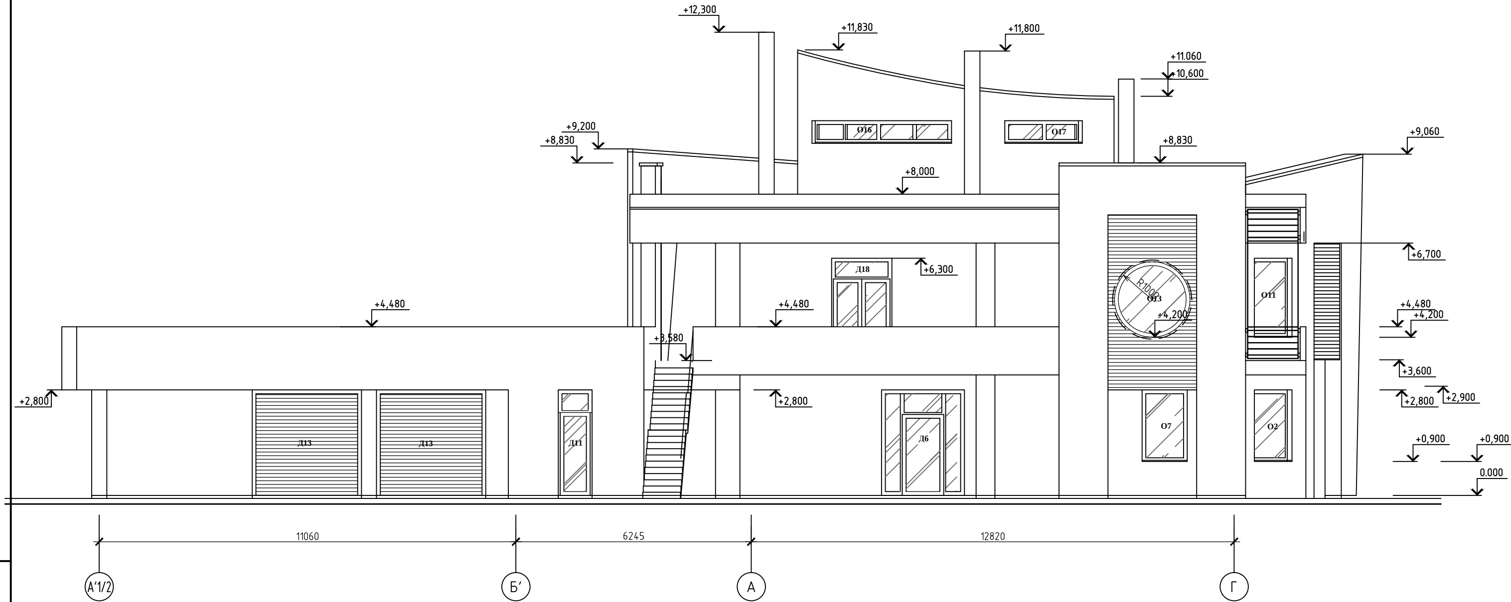
Фасад А-Г М 1:100
